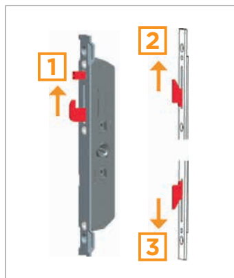
SÉCURITÉ RENFORCÉE Crémone bi-directionnelle à crochets pour maximiser le niveau de sécurité de la baie (3 points pour hauteur ≥ 850 mm).
