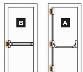
PORTE 1 VANTAIL Barre anti-panique ou push barre 1 point ou 3 points de fermeture.
