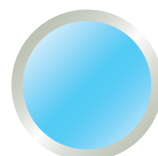
Hublots ABA (2) rond vitrage composite glace PMMA (5) sablé (3) Dimensions (contour extérieur) : Ø 315 mm Ø 235 mm Ø 175 mm Ø 135 mm Ø 105 mm Ø 85 mm
